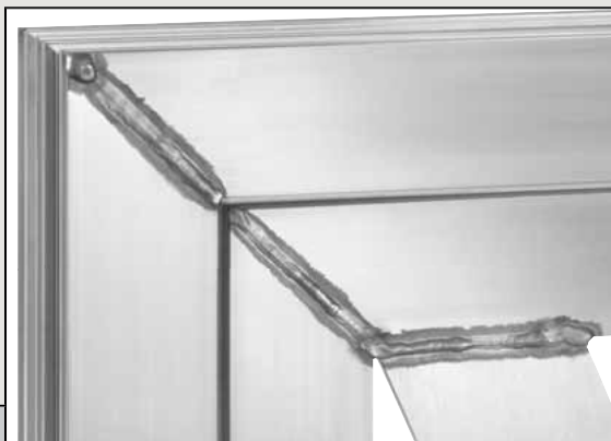
Chaque coupe de profil est soudée manuellement avec précision.
