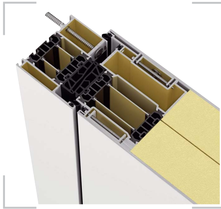
/ Das Profilsystem Therm-105 ist mit reflektierenden Isolier- und Polyamidstegen ausgestattet.
